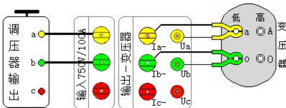
图 25、单相变压器的空载试验
