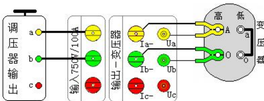
图 27、单相变压器的短路试验
