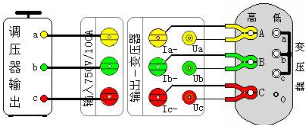
图 28、三相电源对三相变压器短路试验
