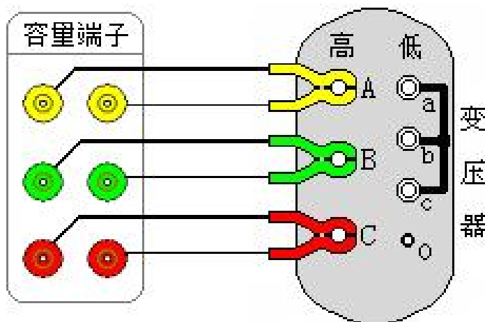
图 24、容量测试接线示意图
