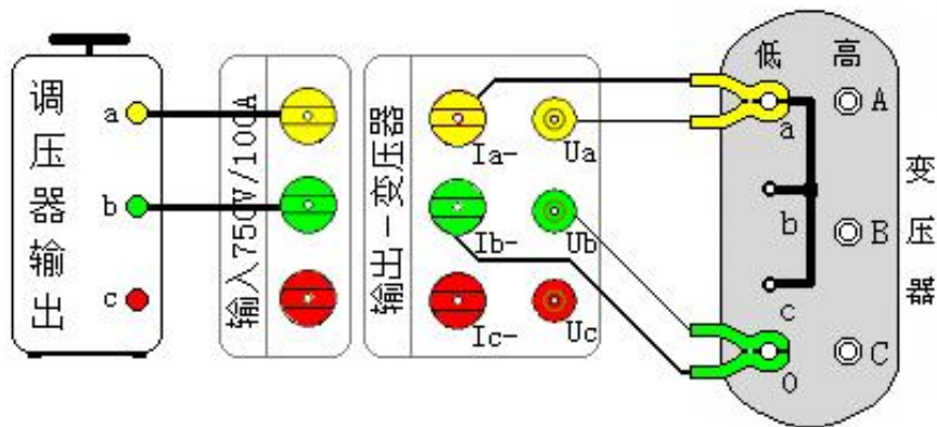
图 29 零序阻抗测试接线
